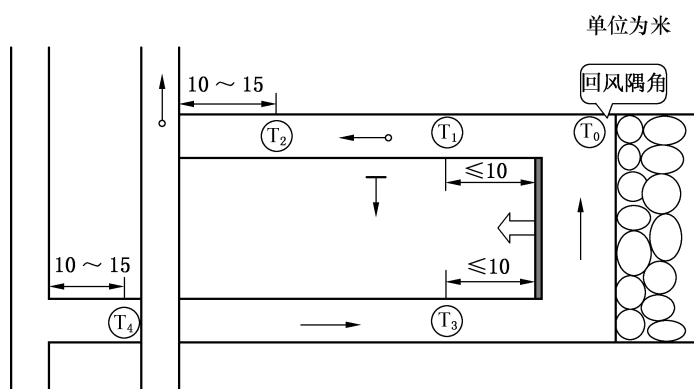
a) U 形通风方式
